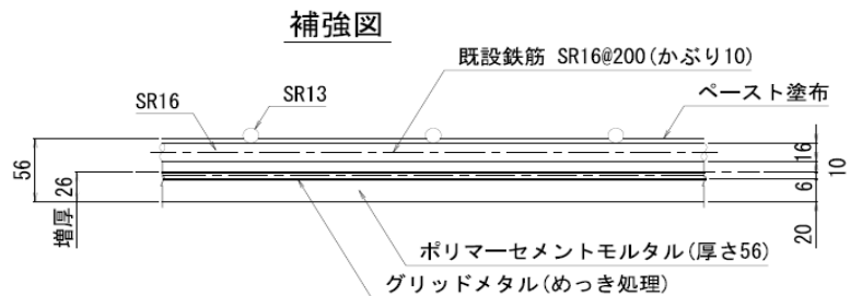
断面図(天井部) S=1:4
